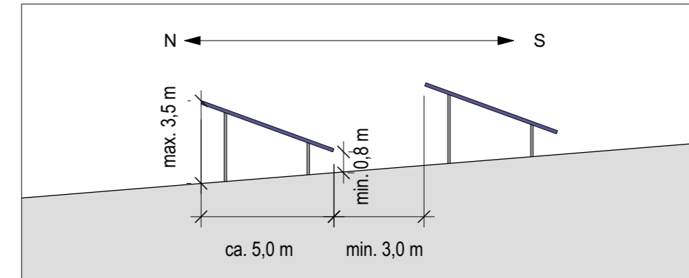
Systemschnitt PV-Trace T1.1 M 1 : 200
